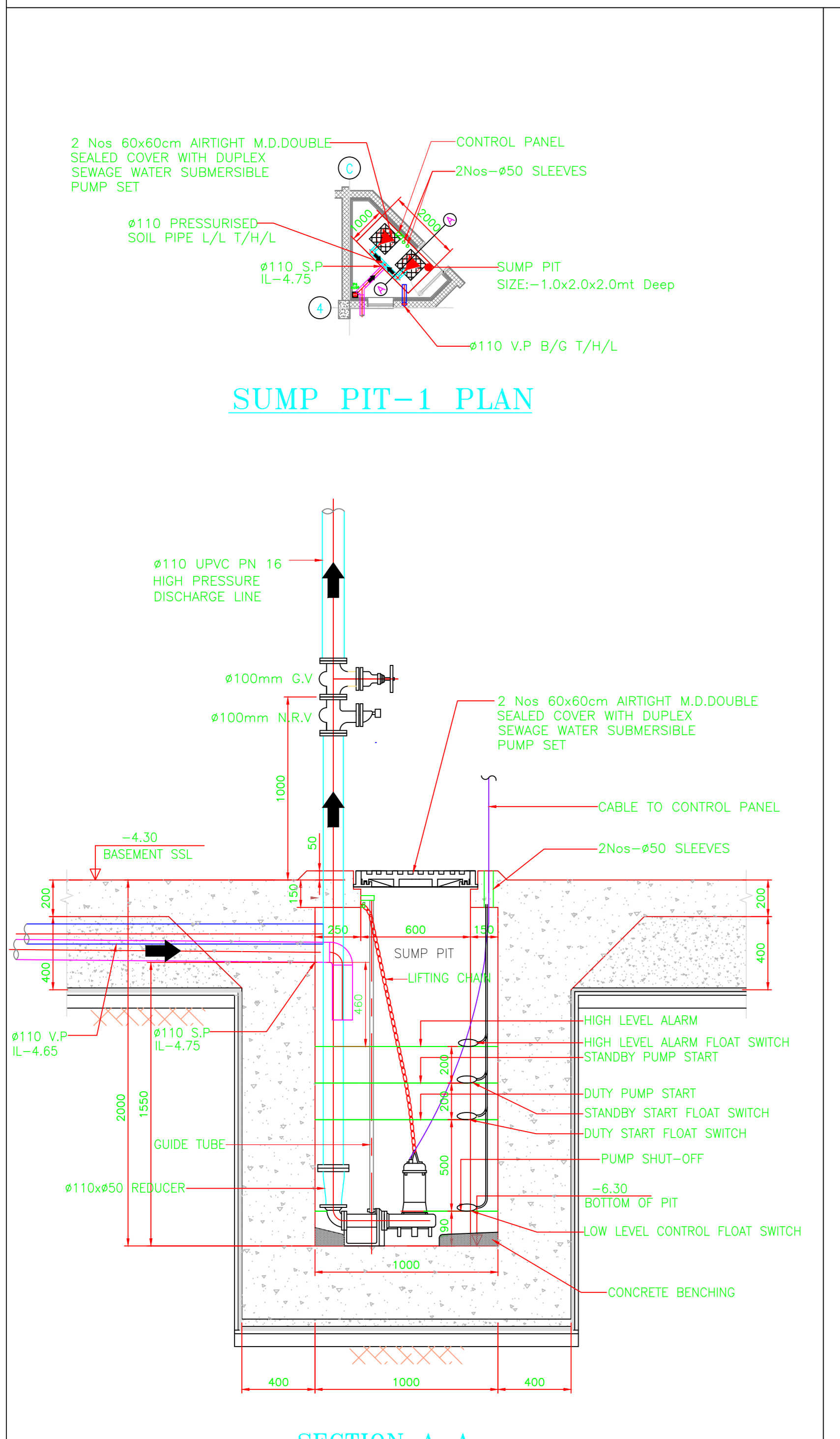
SECTION A-A
