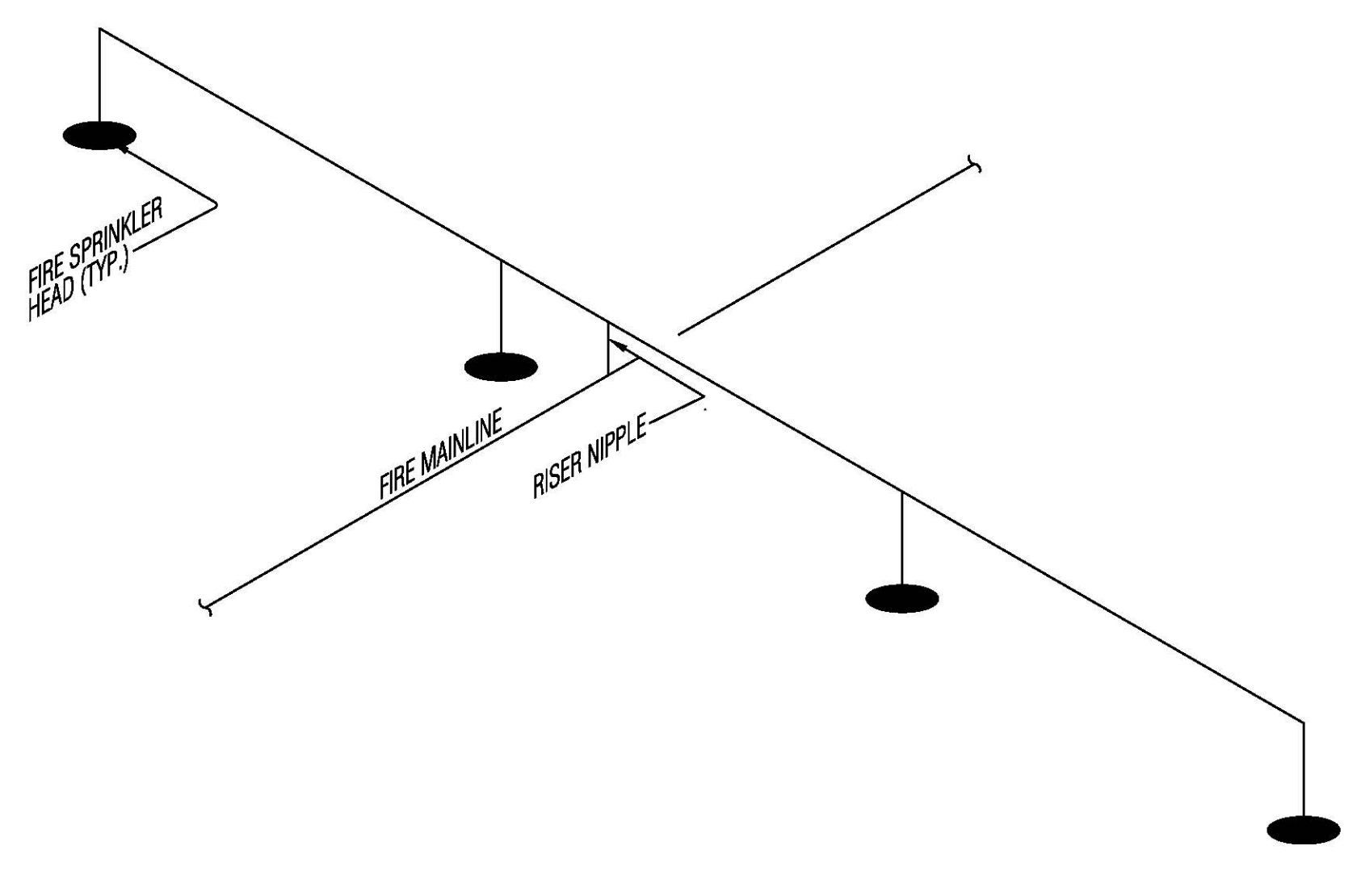
10 FIRE SPRINKLER HEAD G-PP002 N.T.S.
