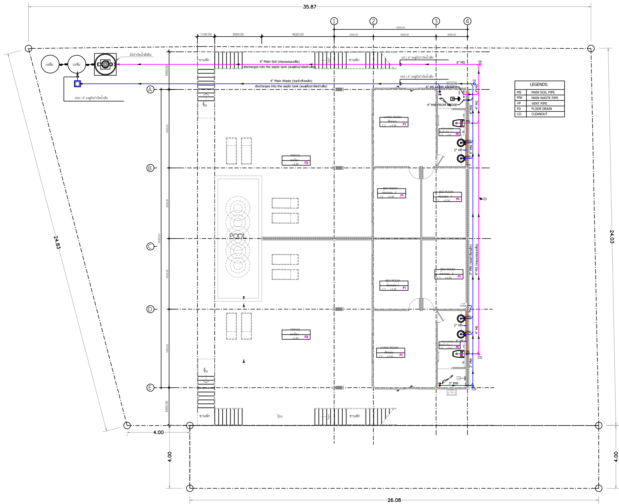
แบบผังสุขาภิบาลชั้น 1 มาตราส่วน 1:125
