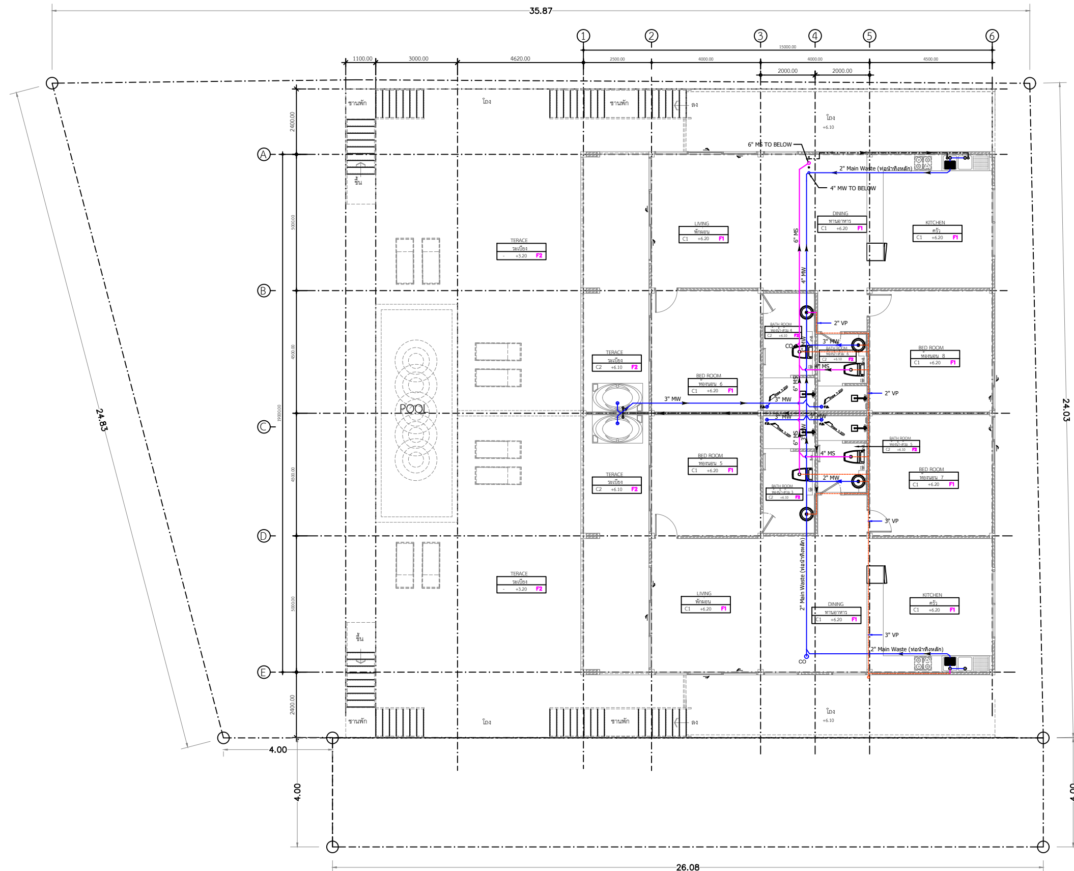
แบบผังสุขาภิบาลชั้น 2 มาตราส่วน 1:125
